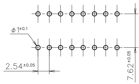
基板穴参考図
